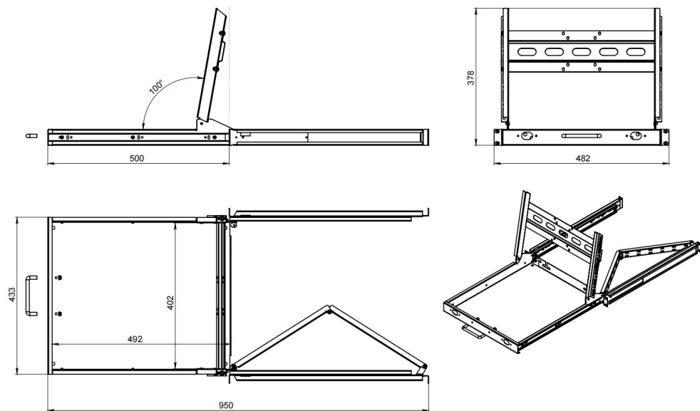
Рисунок 3 - Чертёж полки в рабочем положении
