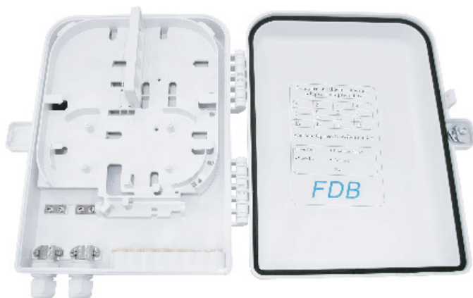
Рисунок 2 - Внутренний конструктив
