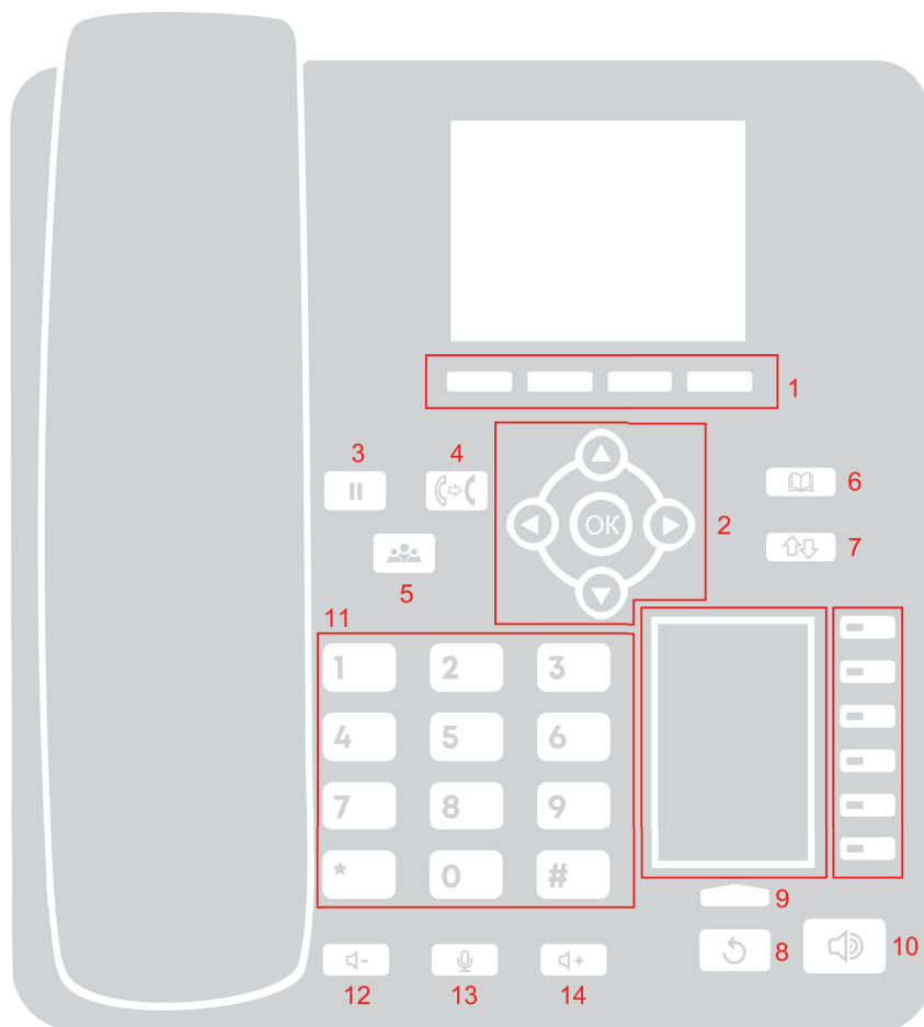
Рис. 4 - Клавиатура
