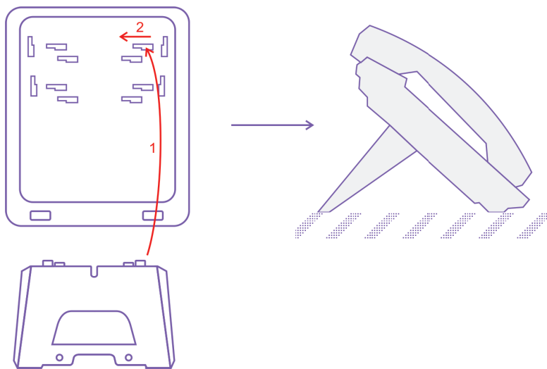
Рис. 1 – Настольное исполнение
