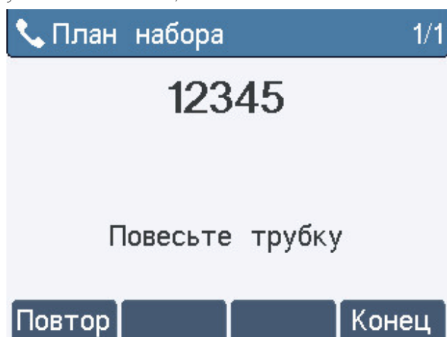
Рис. 34 – Сначала открытие аудио канала, затем набор номера
