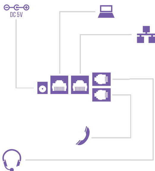
Рис. 3 – Подключение устройства
